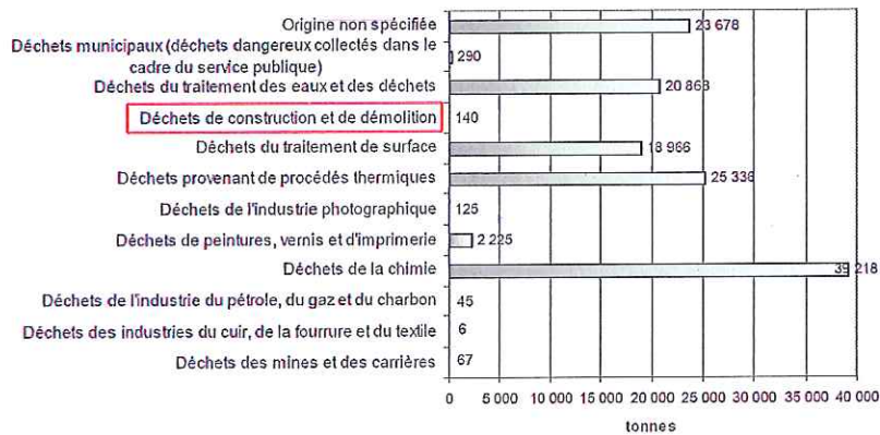
Figure 3 : Activités d'origine des déchets dangereux produits par les gros producteurs – GEREPE 2005
